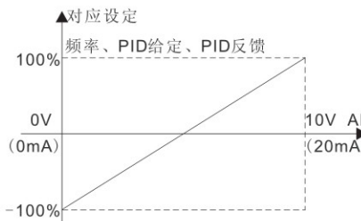
图 6-13 模拟给定与设定量的对应关系
