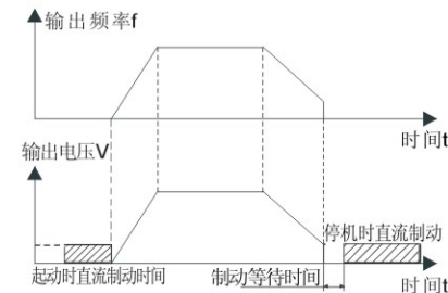
图6-3 直流制动示意图
