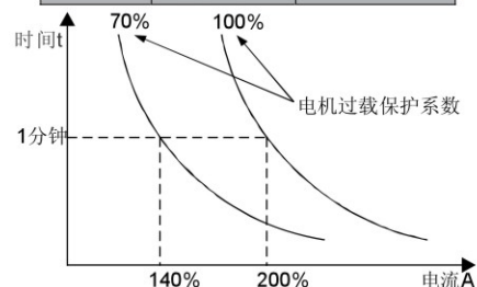
图 6-27 电机过载保护系数设定
