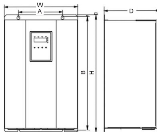
图 A-2 18.5~110kW 机型外形尺寸 (380V)
