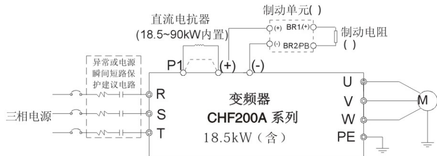
图 4-14 18.5kW
