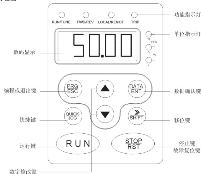
图 5-1 键盘示意图
