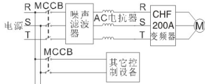
图 4-19 主回路电源侧连接图
