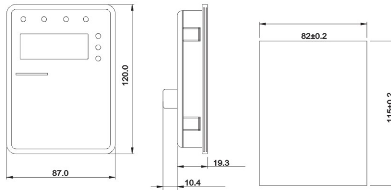
图 A-11 外引键盘（大）的安装尺寸
