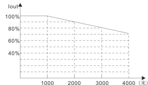
图 3-1 安装海拔高度与变频器降额曲线
