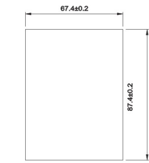
图 A-10 外引键盘（小）的开孔尺寸
