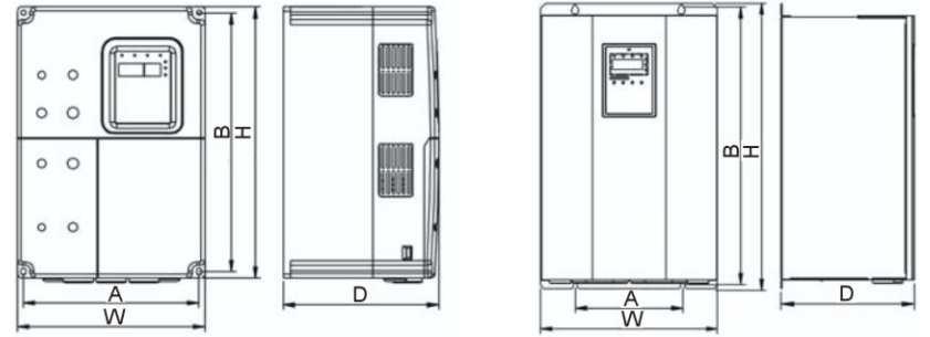
图 A-4 7.5kW 及以下机型的外形尺寸（220V）
