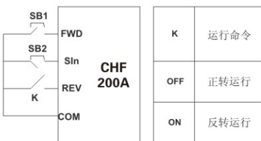
图 6-11 三线式控制模式 1
