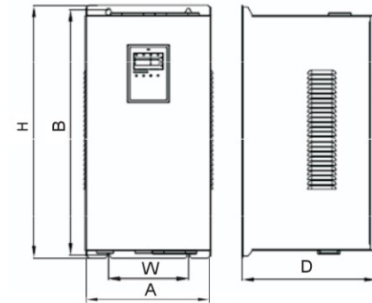
图 A-6 22~55kW 机型的外形尺寸（220V）
