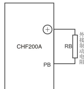
图 B-1 制动电阻的安装
