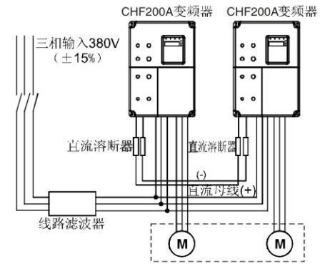
图 4-22 共直流母线的连接
