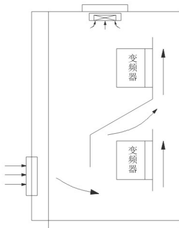
图 A-8 多台变频器的安装
