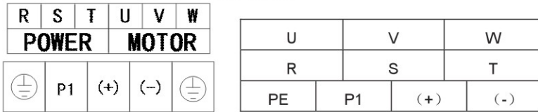
图 4-6 主回路接线端子图 (132~315kW)
