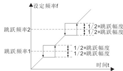
图6-17 跳跃频率示意图
